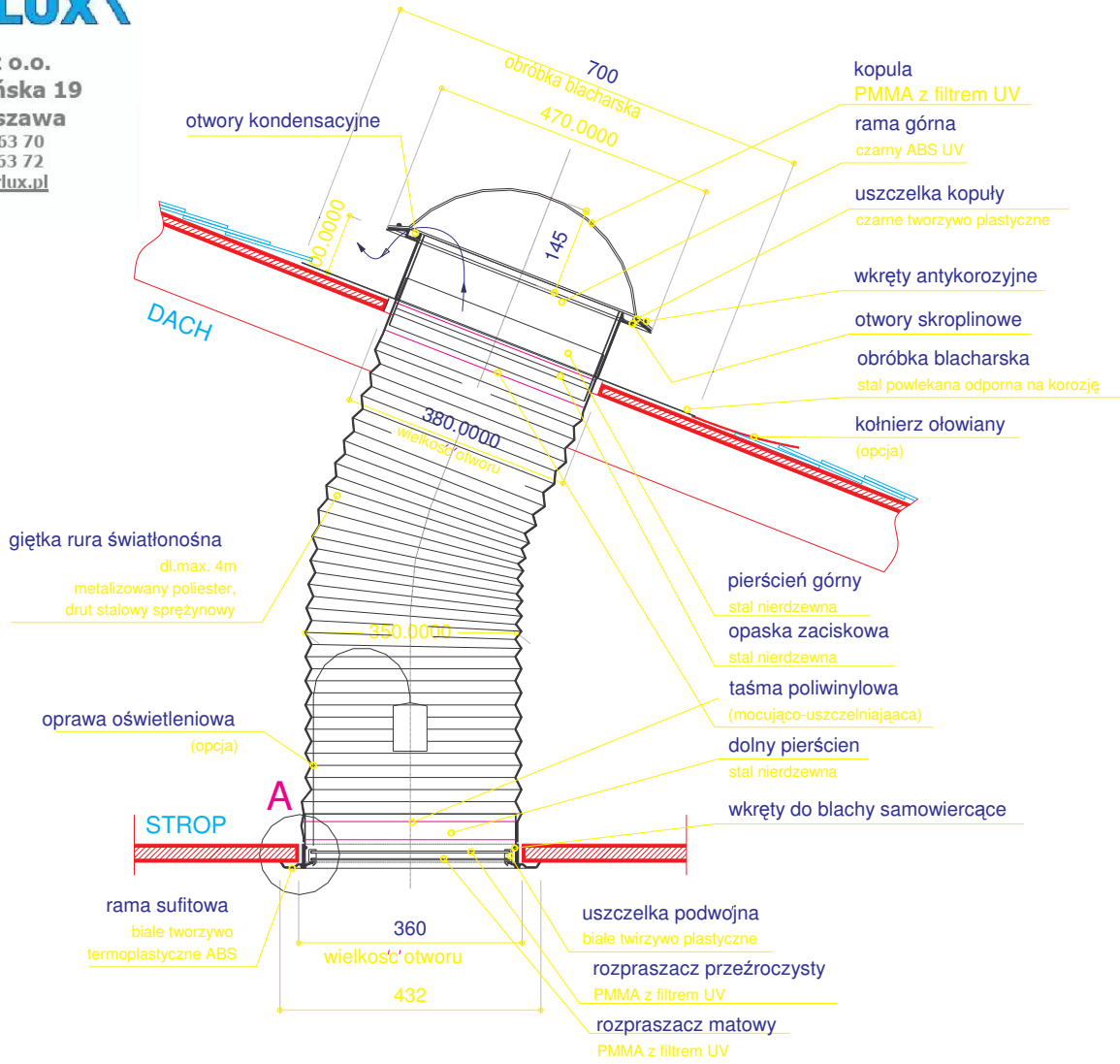
Schemat zestawieniowy elementów światła rurowego maxiSolar® medium
