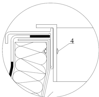
Szczegół A
