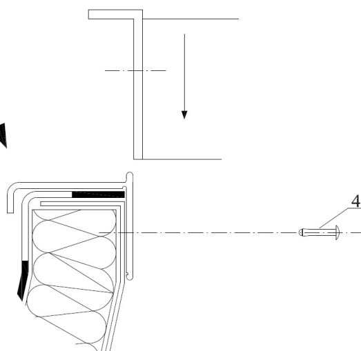
Rys. 8. Montaż napędu klapki dymowej
