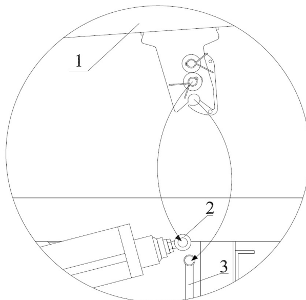
Szczegół B
